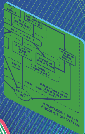
Del av diagram över MYCIN:s informationsflöde
