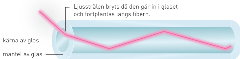
Figur 2. Optisk fiber. En fiber är tunnare än ett hårstrå. Inuti studsar strålen mot gränsen mellan fiberkärnan och manteln då glasets i kärnan har högre optisk täthet än i manteln. Kärnan är cirka 10 mikrometer i diameter, med manteln är fibern 125 mikrometer. Infrarött ljus med en våglängd på 1,55 mikrometer, där ljusförlusterna är lägst, används idag för långväga fiberoptisk kommunikation.
